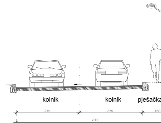
POPREČNI PRESJEK ZA OSTALE ULICE OZNAKE "B" I "C" (DVOUSMJERNI PROMET)
