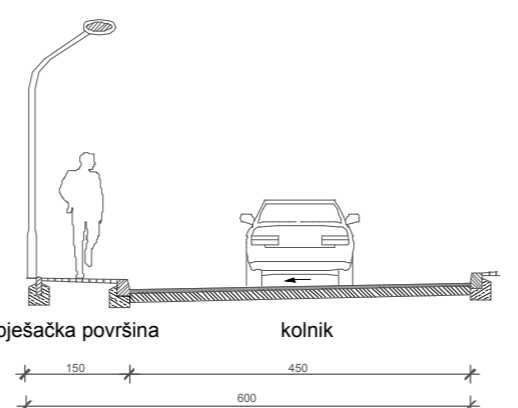
POPREČNI PRESJEK ZA OŠTALU ULICU OZNAKE "A" (JEDNOSMJERNI PROMET)
