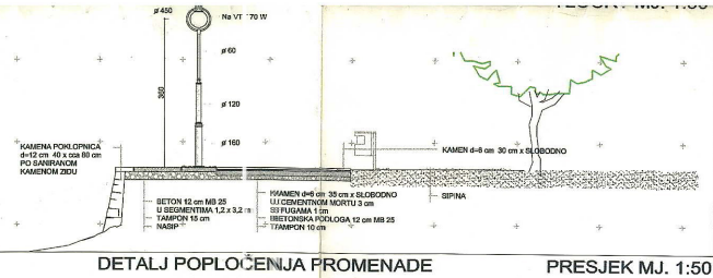
DETAILJ POPLOČENJA PROMENADE PRESJEK MJ. 1:50
