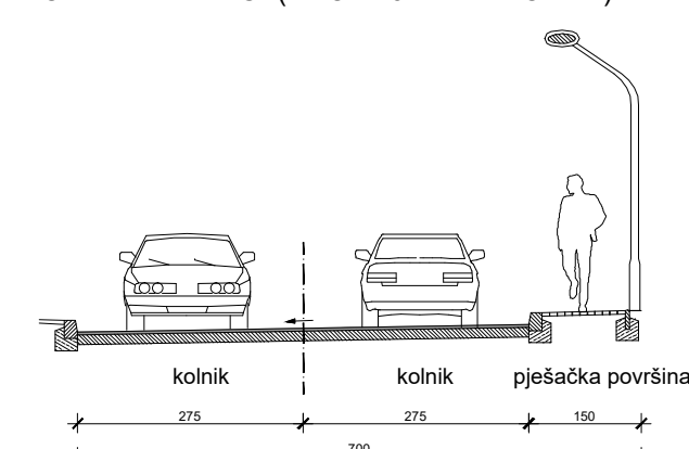
POPREČNI PRESJEK ZA OSTALE ULICE OZNAKE "B" I "C" (DVOUSMJERNI PROMET)
