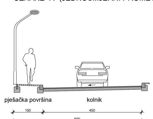
POPREČNI PRESJEK ZA OSTALU ULICU OZNAKE "A" (JEDNOSMJERNI PROMET)
